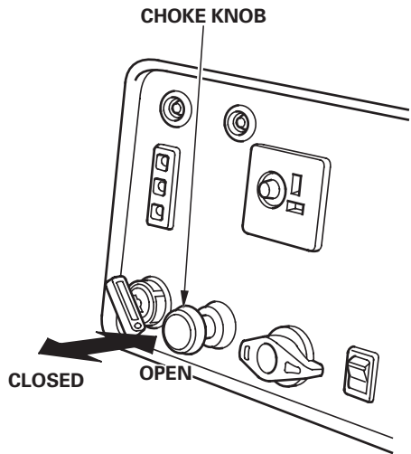
CHOKE KNOB
